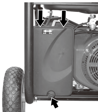
Монтаж на капака на въздушния филтър
